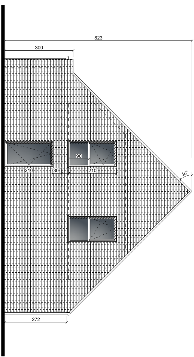
Pignon (Sud)
